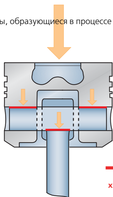
Распределение сил в поршне и шатуне при сопряжении прямоугольной формы
