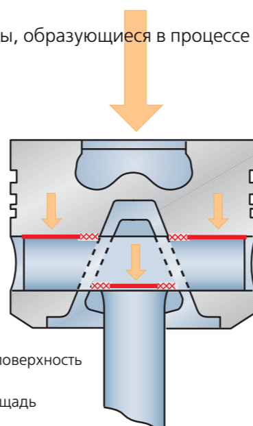
Распределение сил в поршне и шатуне при сопряжении трапецевидной формы
