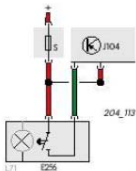
Электронное подключение
