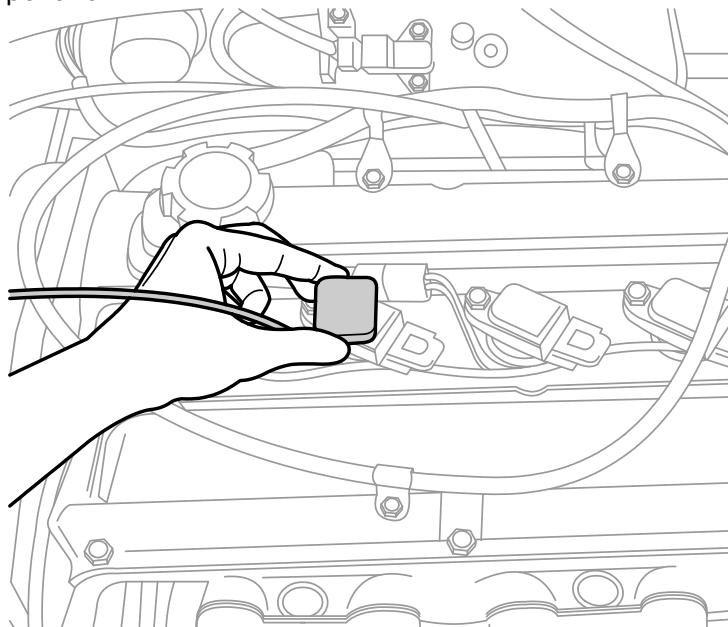
Подключение датчика СОР к катушке зажигания
