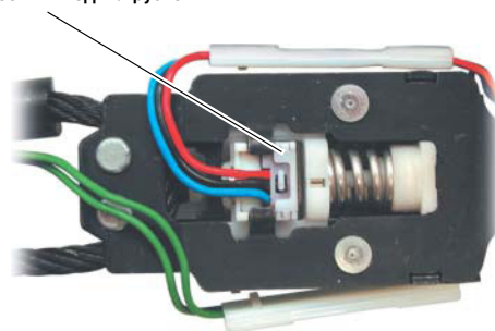
Датчик силы натяжения ремня безопасности – под нагрузкой
