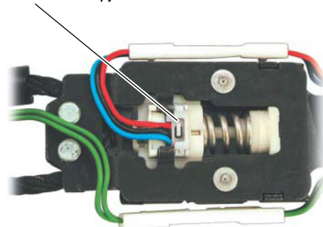
Датчик силы натяжения ремня безопасности – без нагрузки
