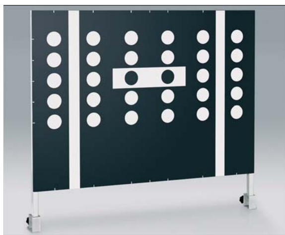
VAS 6430/4 калибровочный экран ассистента движения по полосе
