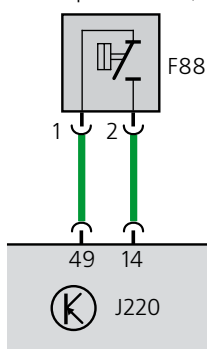
Электрическая цепь
