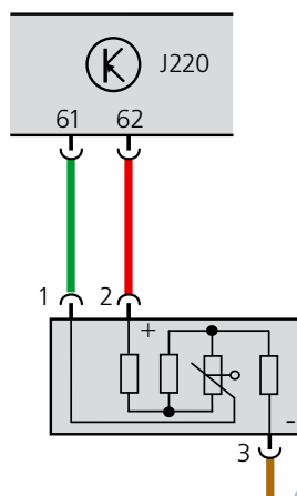
Электрическая цепь
