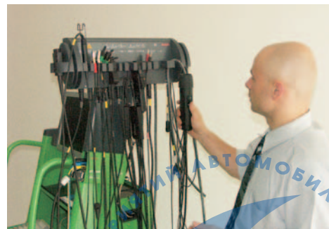
Измерительный модуль FSA 720 представляет собой совокупность полного комплекта датчиков и аналогово-цифрового преобразователя. Это позволяет использовать его в качестве эффективного инструмента моторной диагностики и базового устройства интегрированной диагностической системы.
