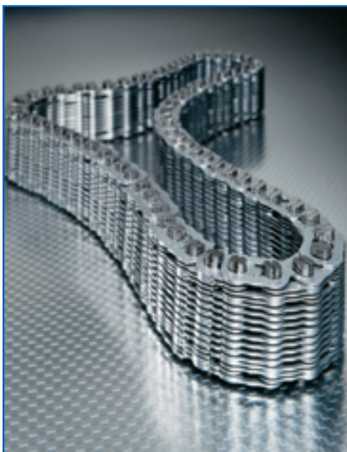
В «мультиатриках» в качестве гибкого элемента вариаторной передачи используется многорядная маложужащая цепь.
