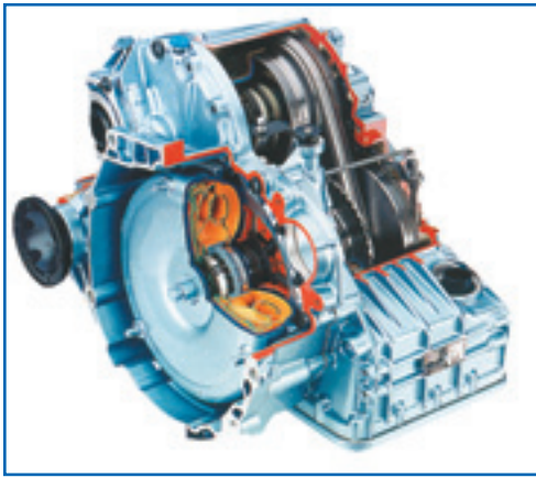
Другая модель ZF Ecotronic рассчитана на трансформацию большего крутящего момента. В ней в качестве узла сцепления с двигателем используется гидротрансформатор.
