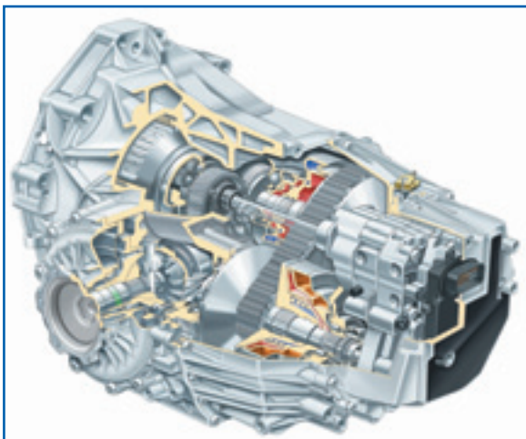
Дебютировав, трансмиссия Multitronic сразу установила рекорд. Ею оснащалась модель Audi A6 с двигателем 2,8 V6 (193 л.с.), развивающим крутящий момент до 280 Н·м.
