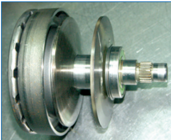
Шкив вариатора состоит из двух конических дисков. Тот, что слева — подвижный, его положение регулируется гидроцилиндром.
