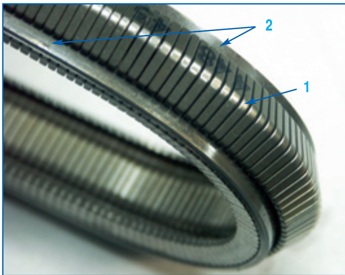
Толкающий ремень сформирован из стальных пластин трапецевидной формы (1), прочно стянутых в замкнутый пакет двумя многослойными металлическими лентами (2).
